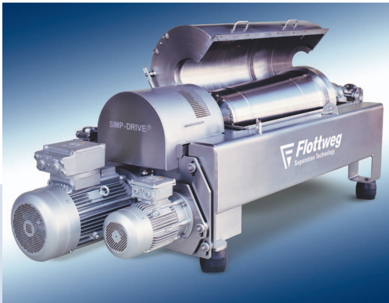
СЕДИКАНТЕР FLOTTWEG S4E-3
