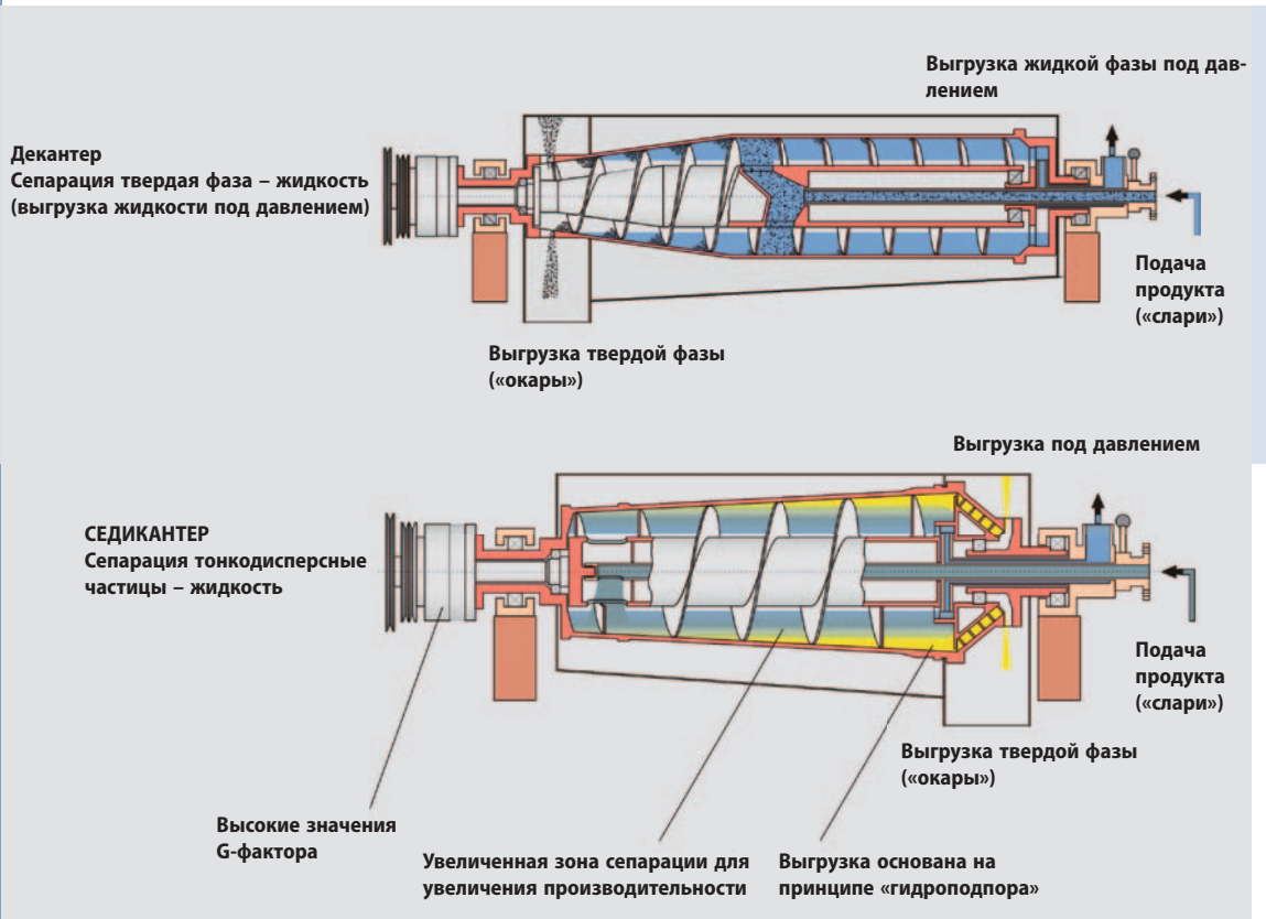
Сравнение СЕДИКАНТЕРА и ДЕКАНТЕРА FLOTTWEG
