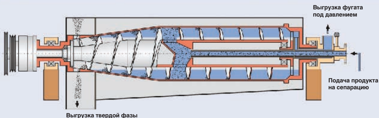
Декантер FLOTTWEG с выгрузкой фугата по давлением
